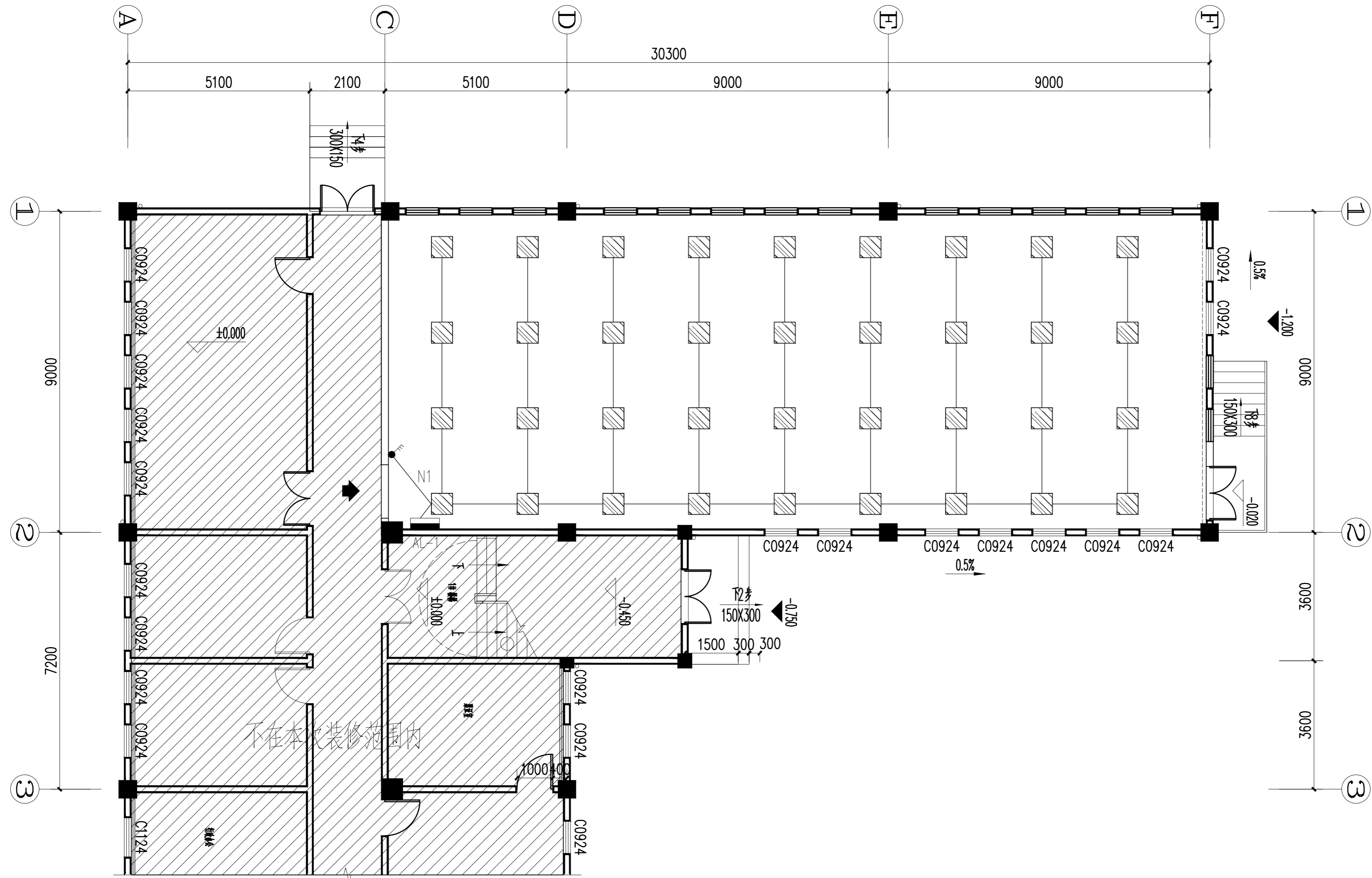
综合楼一层档案室照明线路图
