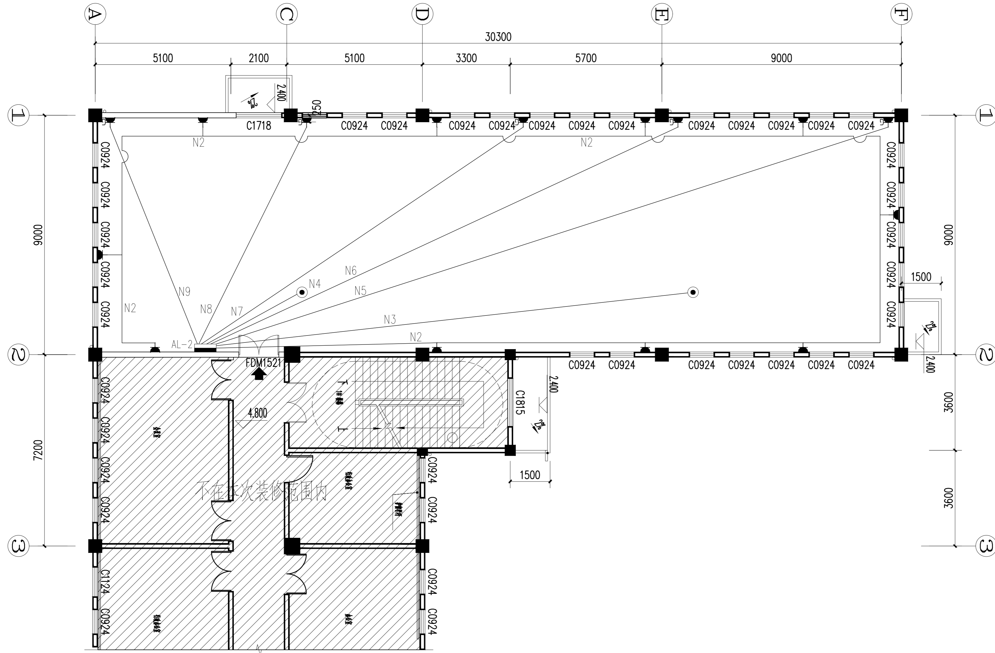
综合楼二层档案室强电插座布置图
