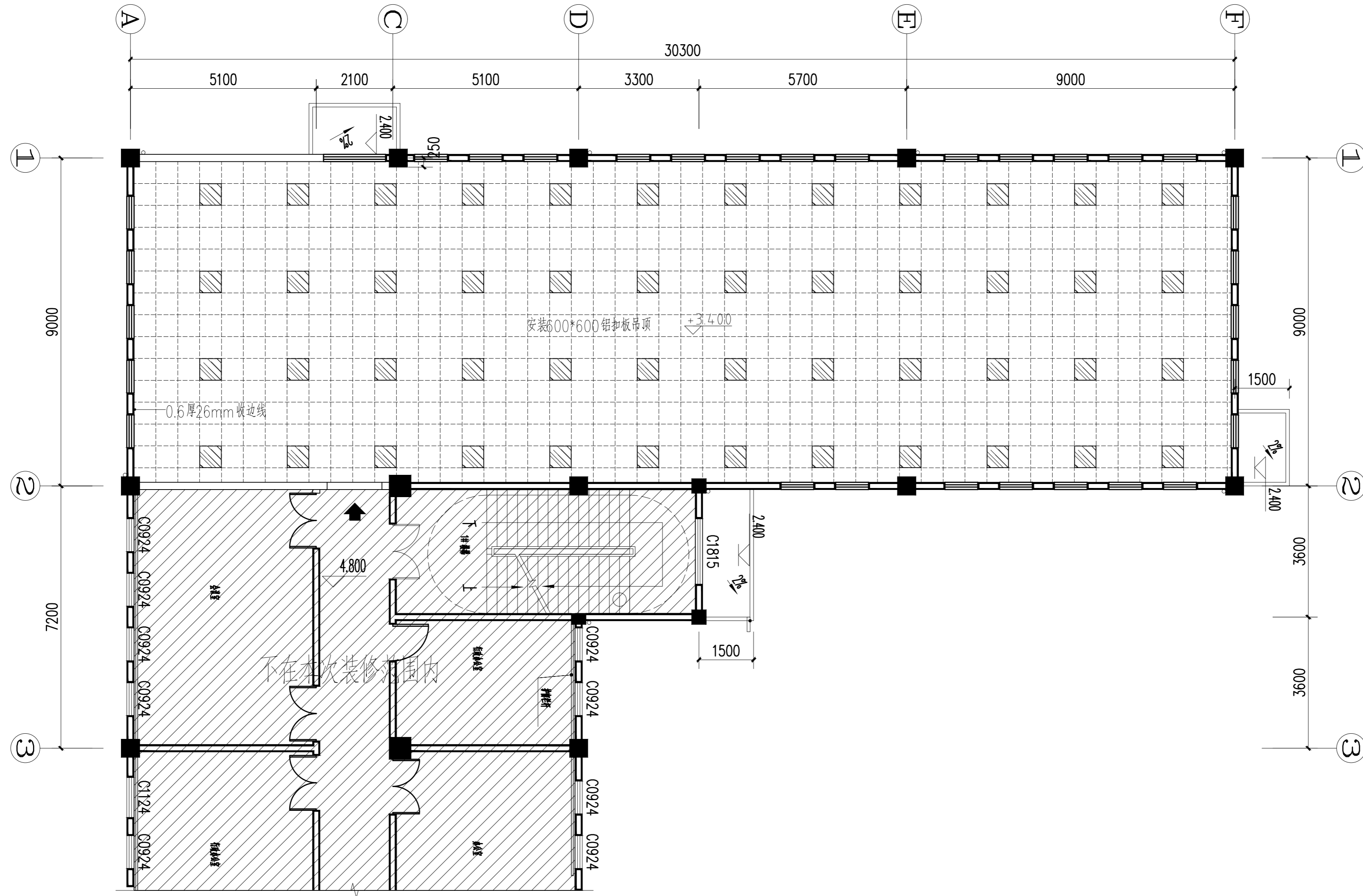
综合楼二层档案室吊顶结构图
