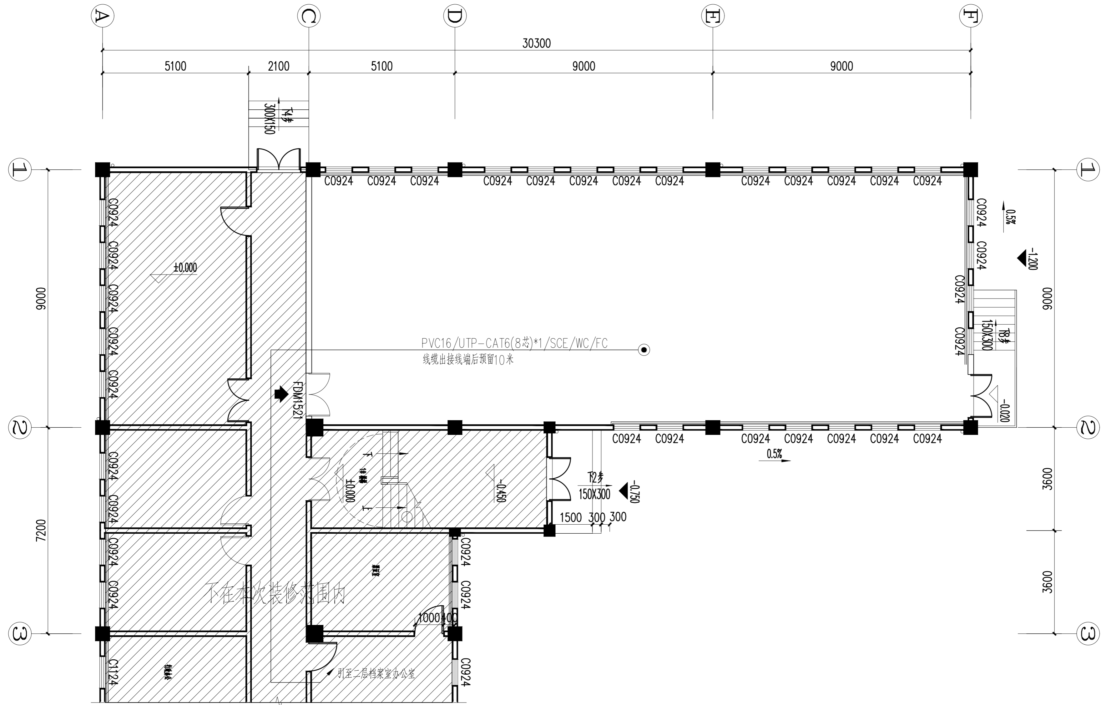
综合楼一层档案室弱电插座布置图
