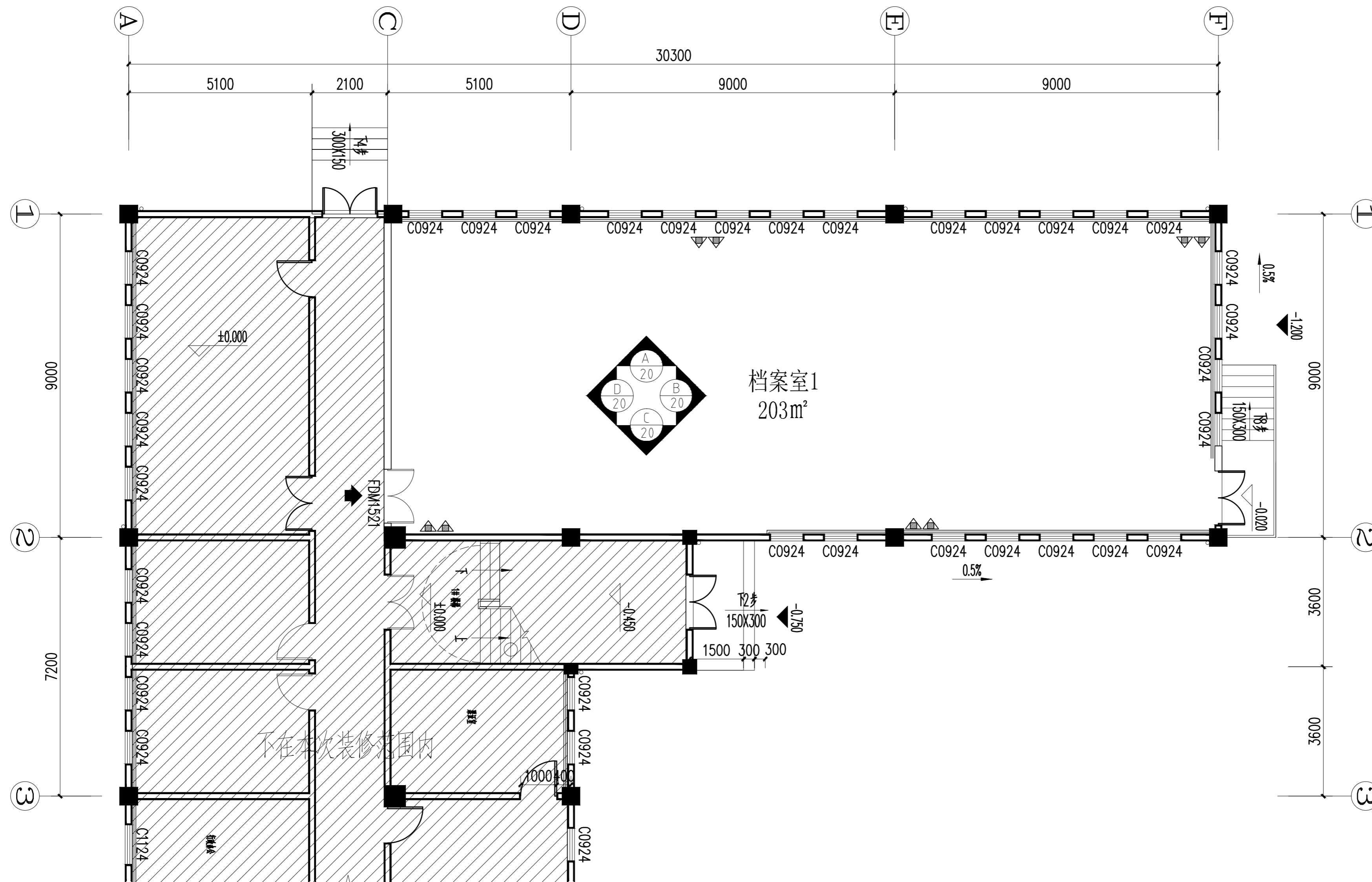
综合楼一层档案室平面图
