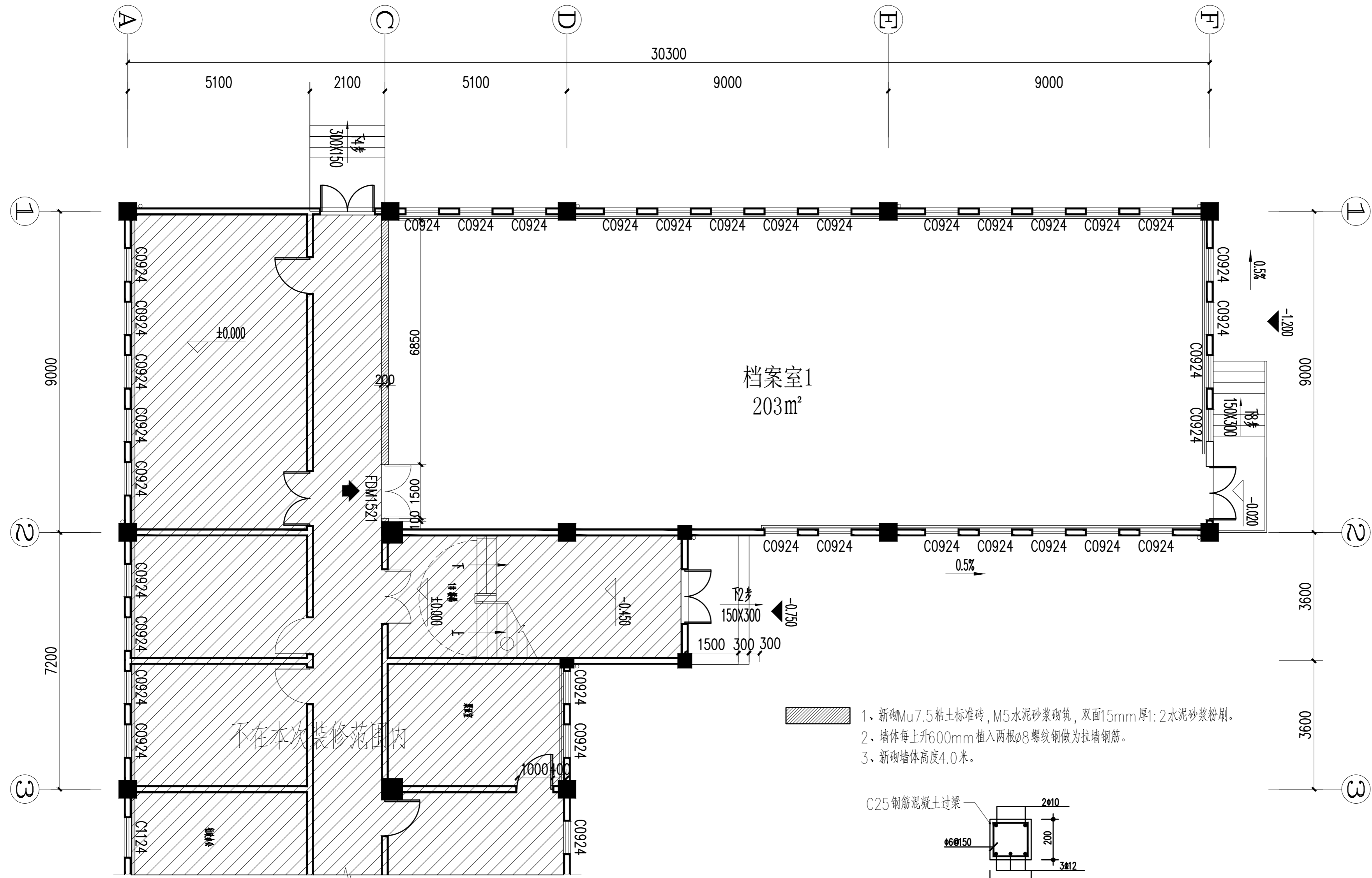
综合楼一层档案室墙体定位图
