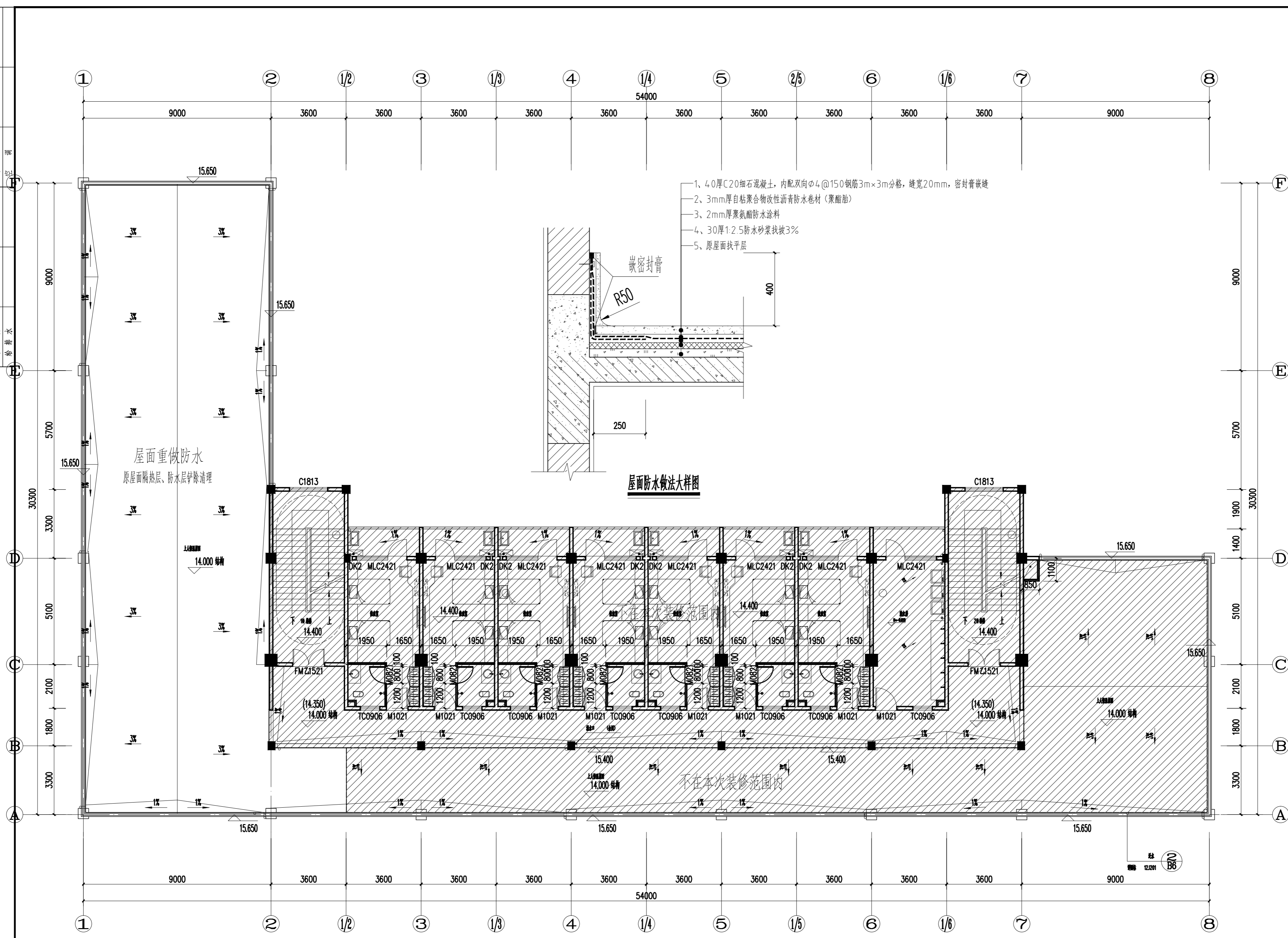
综合楼屋面平面图 1:180
