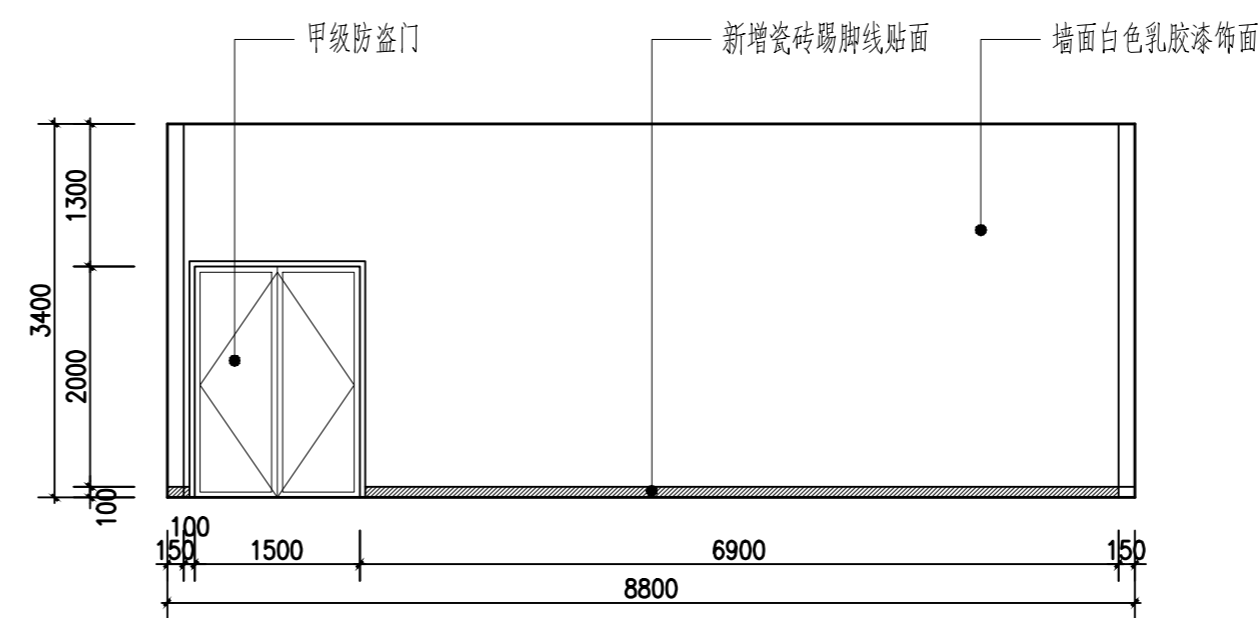
综合楼一层档案室D立面图
