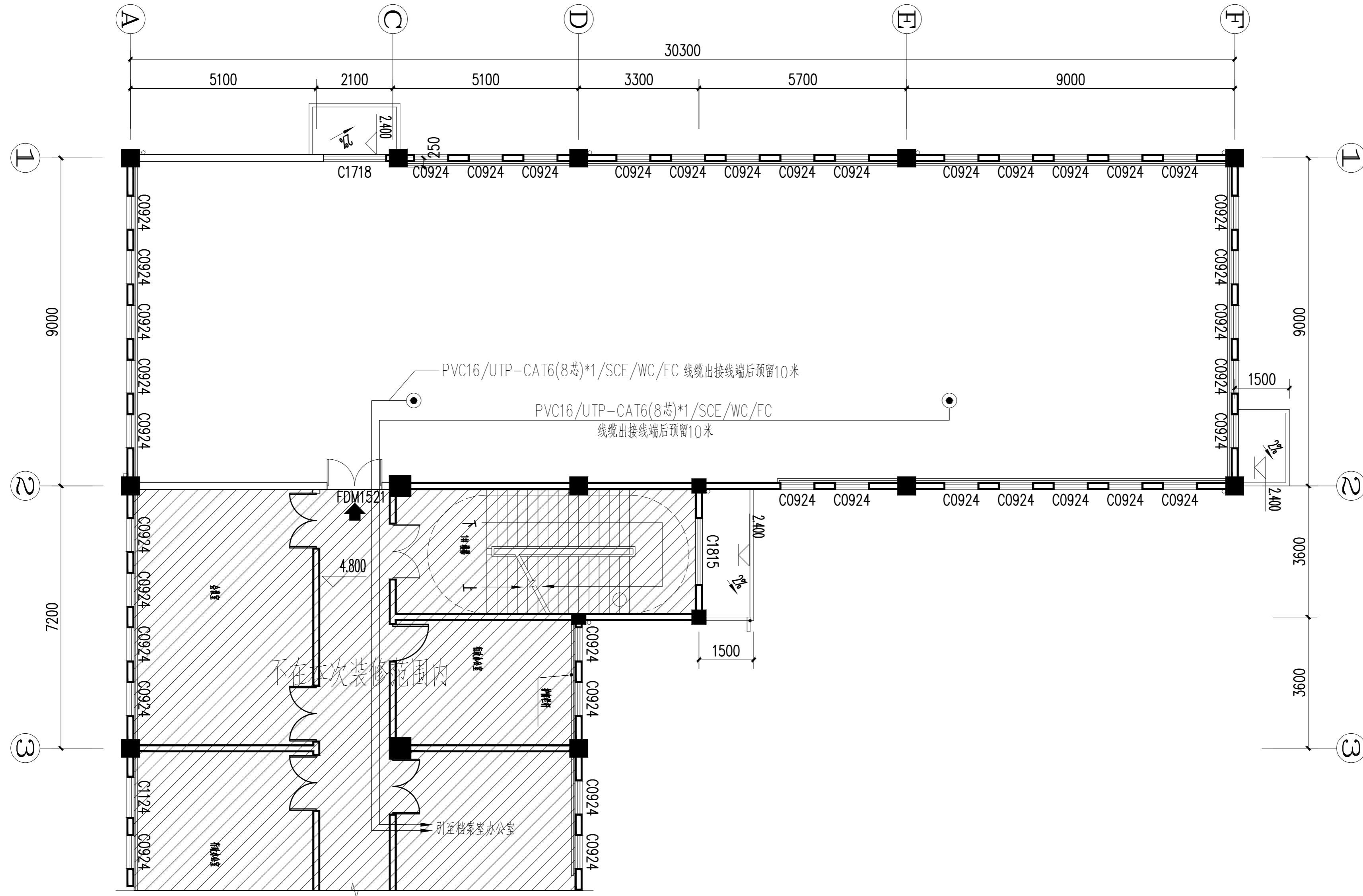
综合楼二层档案室弱电插座布置图
