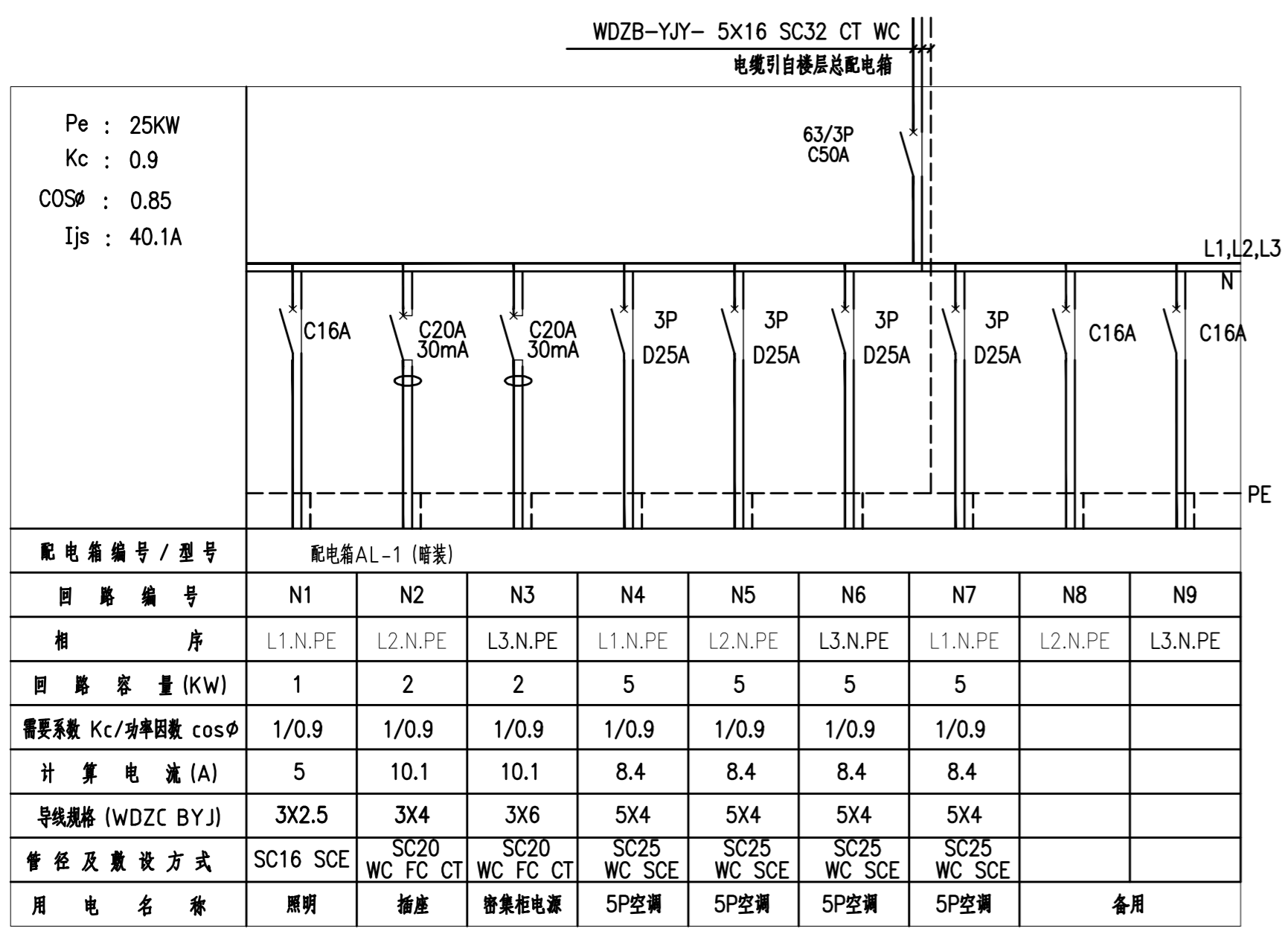
AL-1 配电箱系统图
