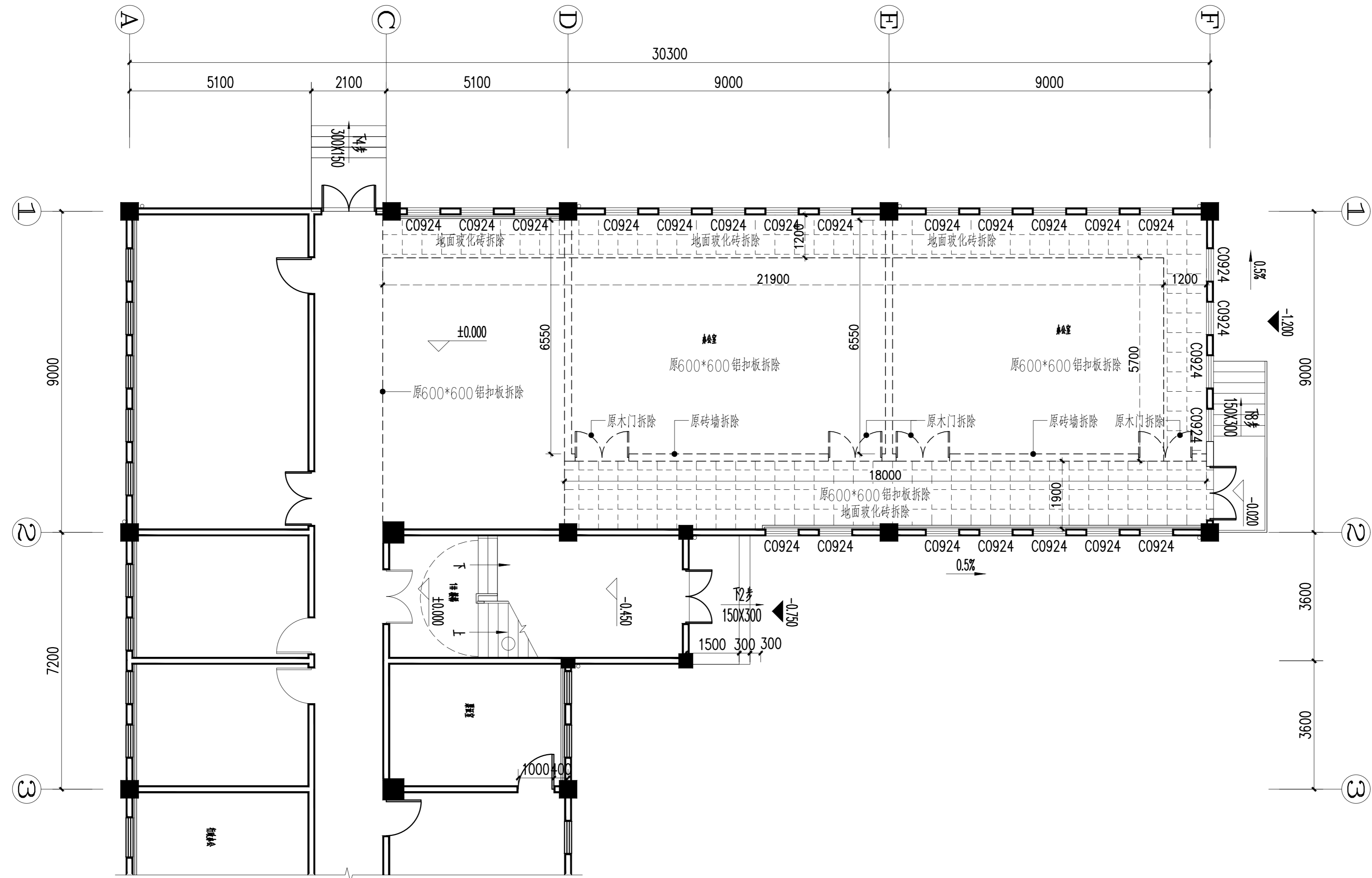
综合楼一层档案室拆除定位图
