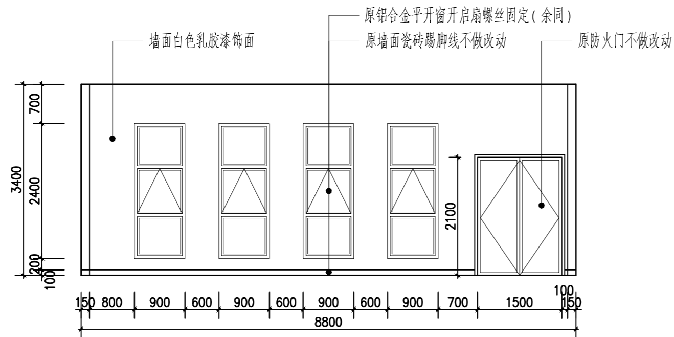
综合楼一层档案室B立面图
