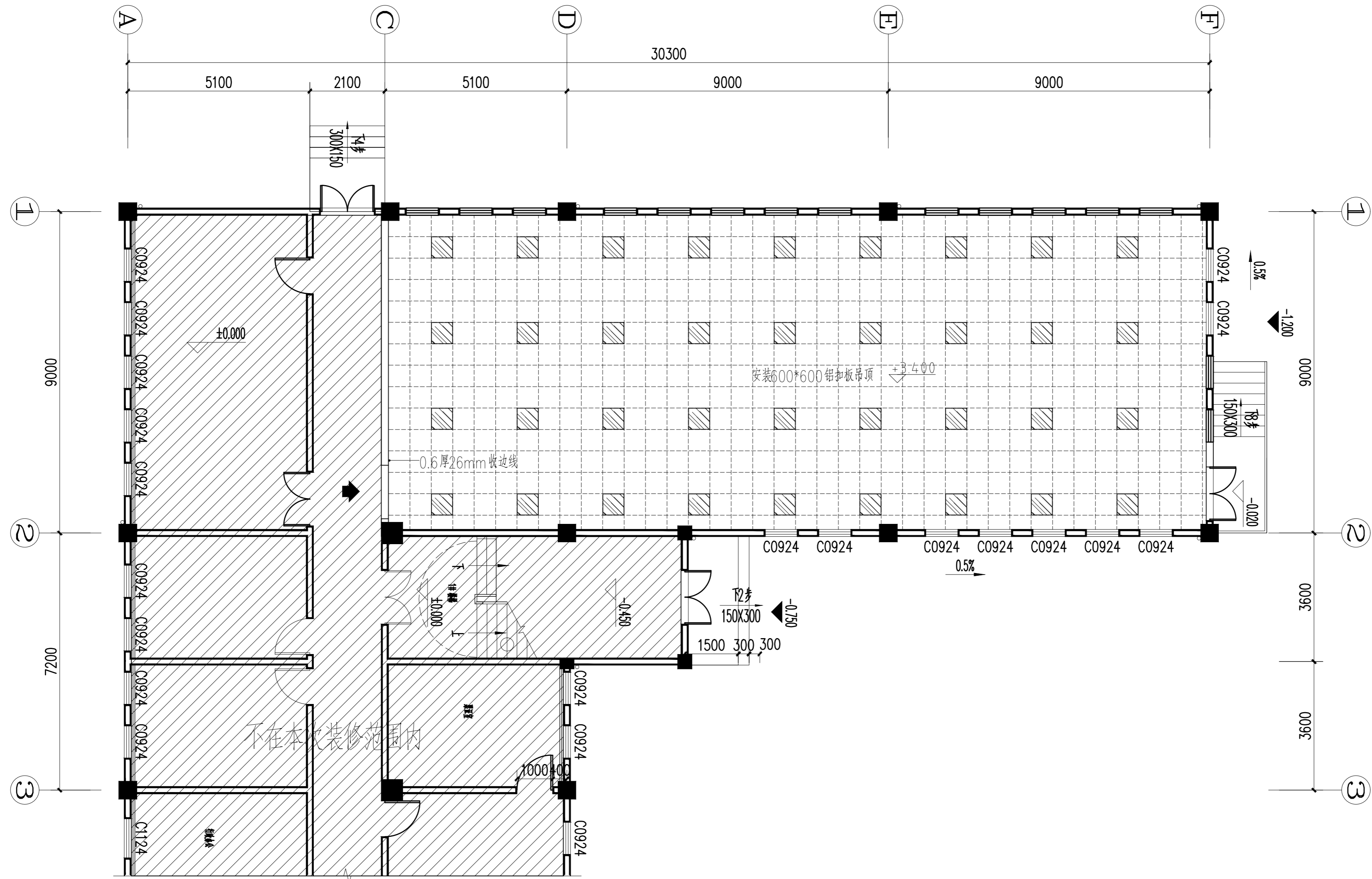
综合楼一层档案室吊顶结构图
