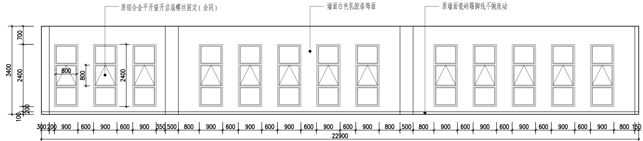
综合楼一层档案室A立面图
