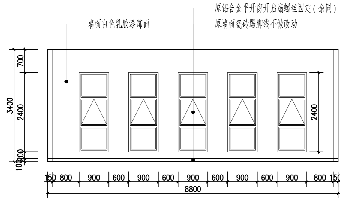
综合楼二层档案室B立面图
