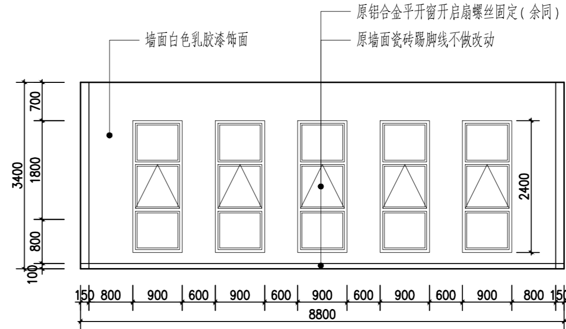
综合楼二层档案室D立面图
