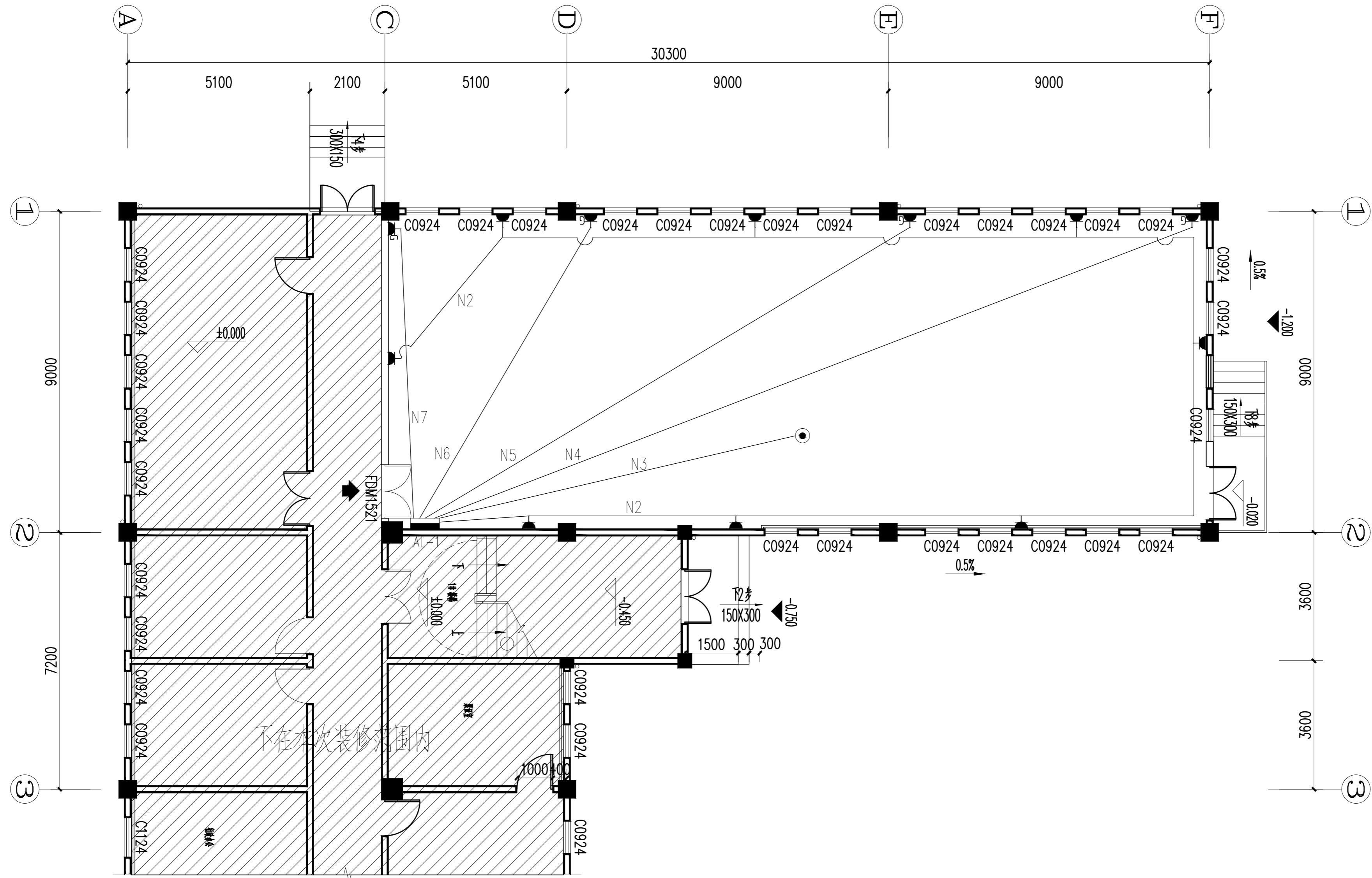
综合楼一层档案室强电插座布置图
