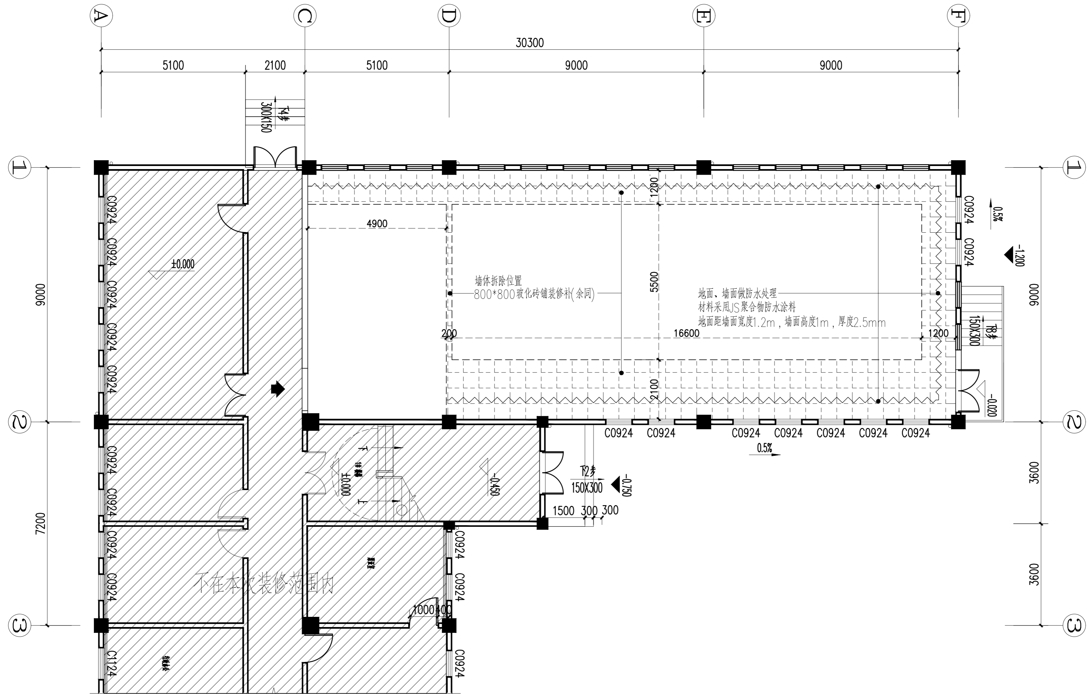
综合楼一层档案室地面铺装图
