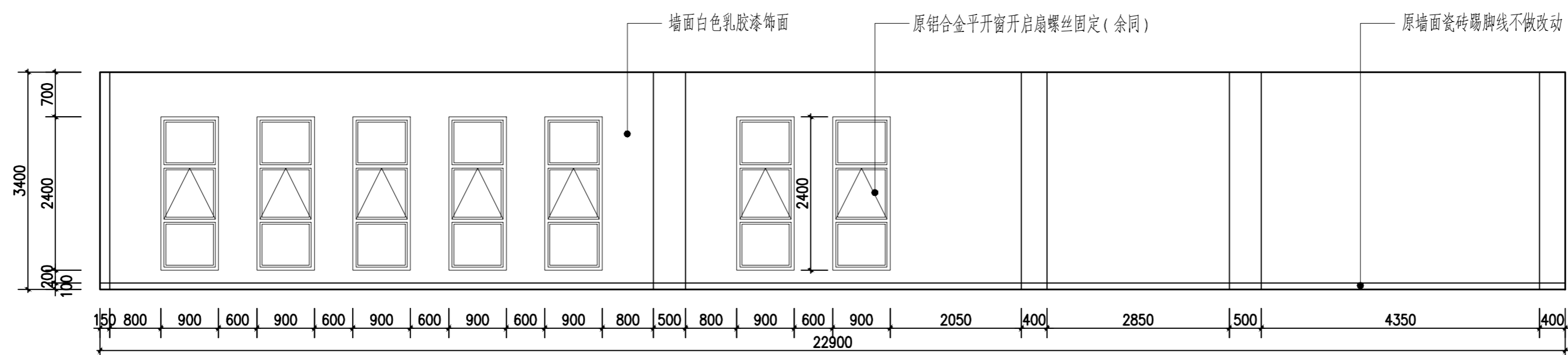
综合楼一层档案室C立面图
