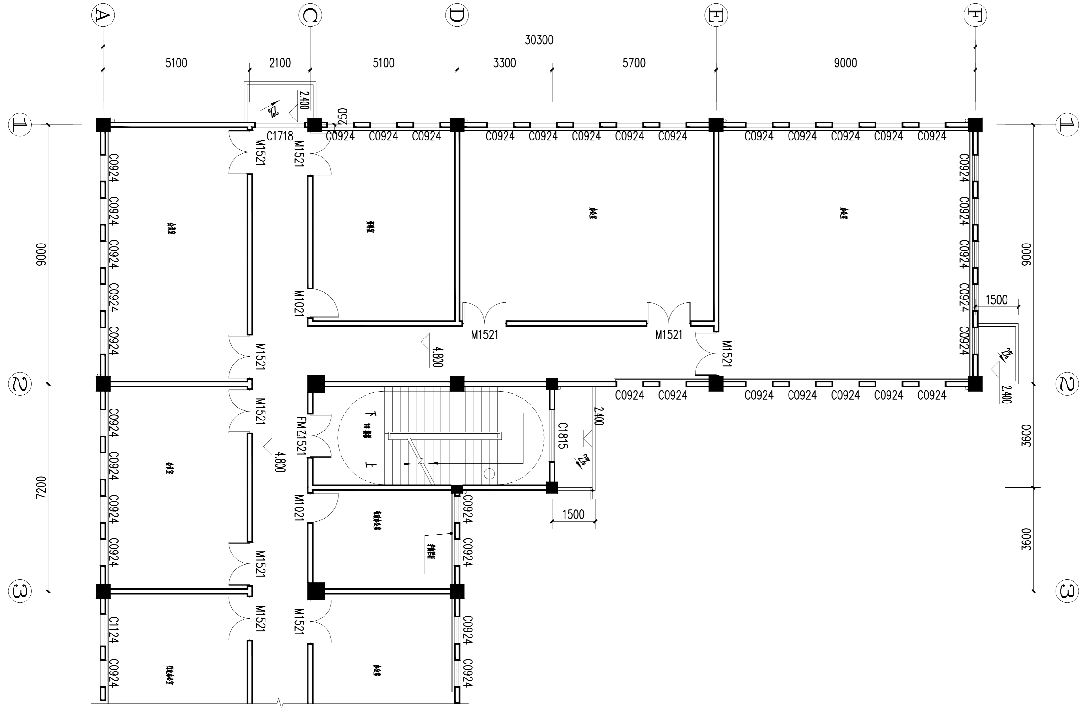
综合楼二层档案室原始结构图
