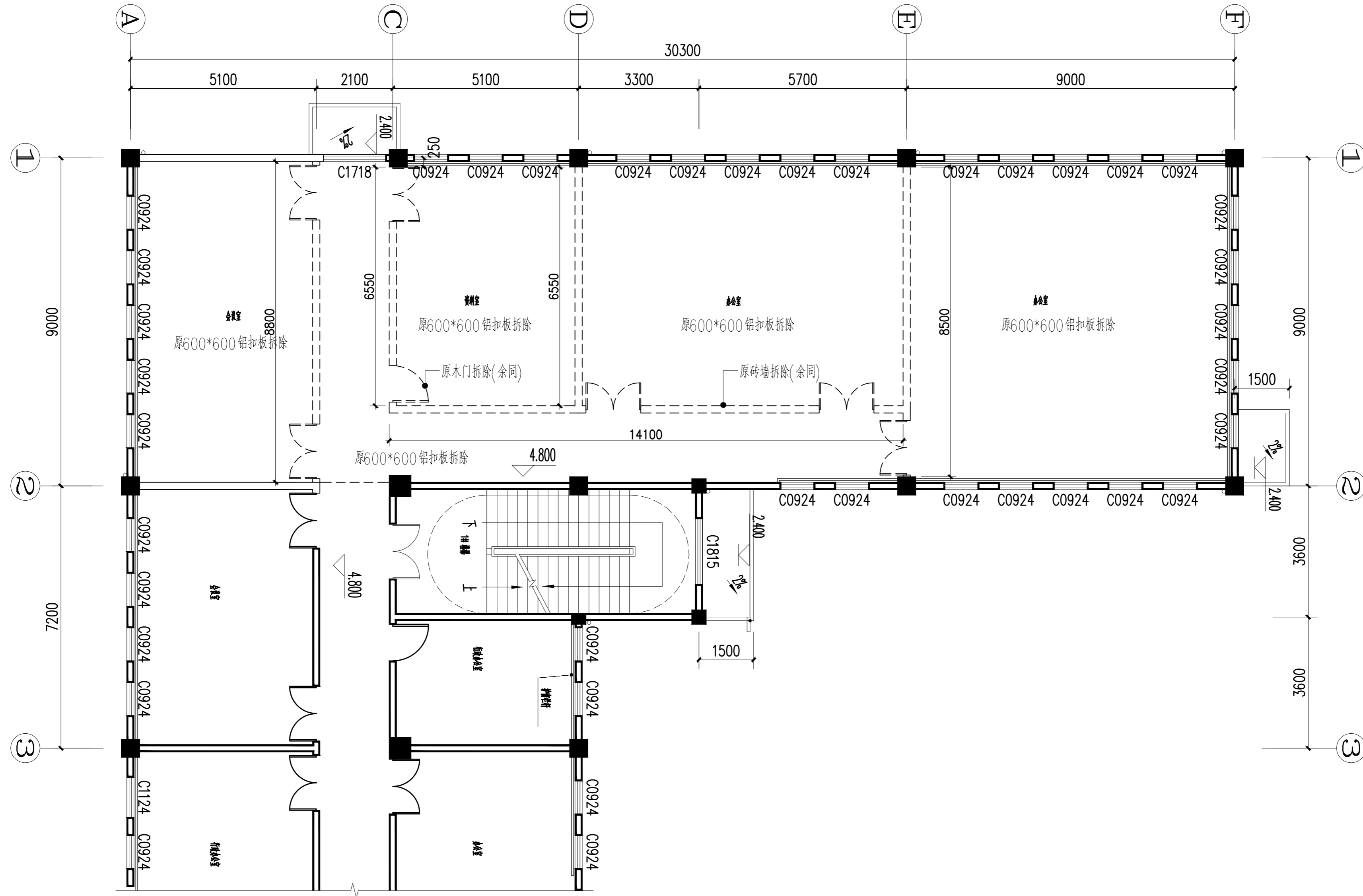
综合楼二层档案室拆除定位图
