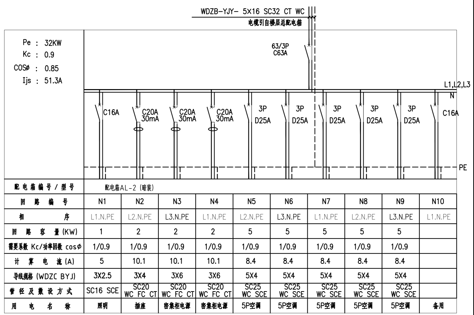
AL-2 配电箱系统图
